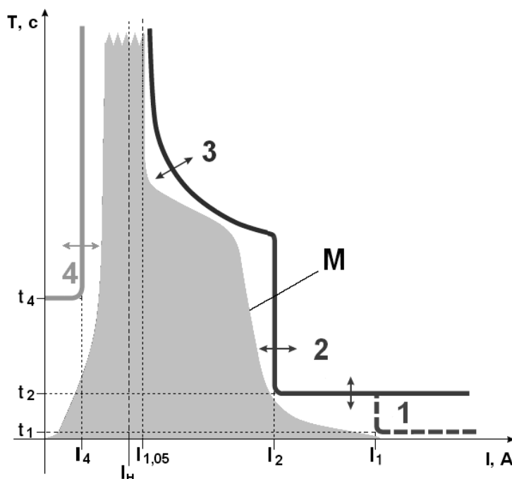
Рисунок 5 – Токвременная характеристика
