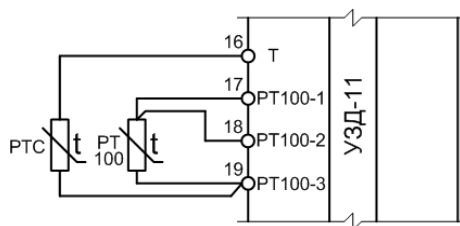
Рисунок 6 – Использование независимого расцепителя для организации быстросрабатывающей защиты от короткого замыкания.
