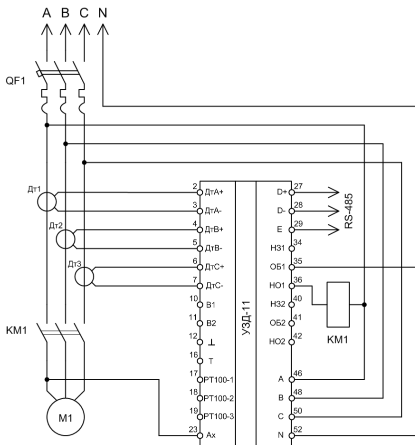
Рисунок 5 – Типовая схема включения: KM1 – магнитный пускатель; QF1 – автоматический выключатель; Дт1, Дт2, Дт3 – датчики тока.
