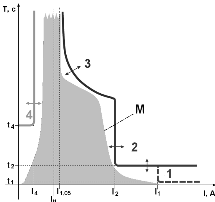
Рисунок 4 - Токременная характеристика
