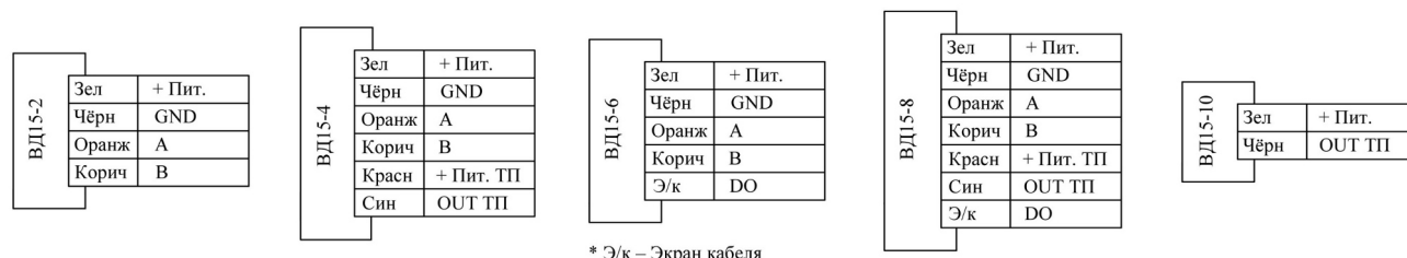
Рисунок 1. Варианты исполнения и подключения датчика ВД15
