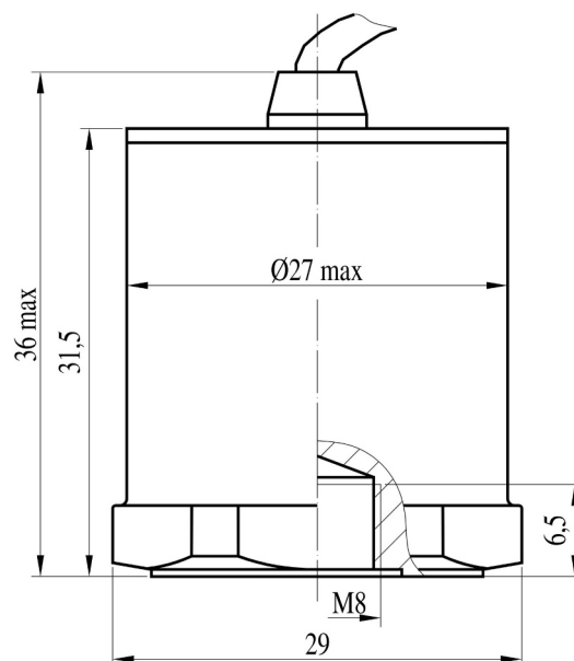
Рисунок 4. Габариты датчика
