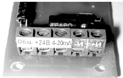
Рисунок 7. Расположение клемм для подключения проводов
