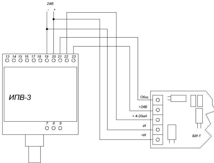
Рисунок 4. Подключение БИ-1 к преобразователю ИПВ-3
