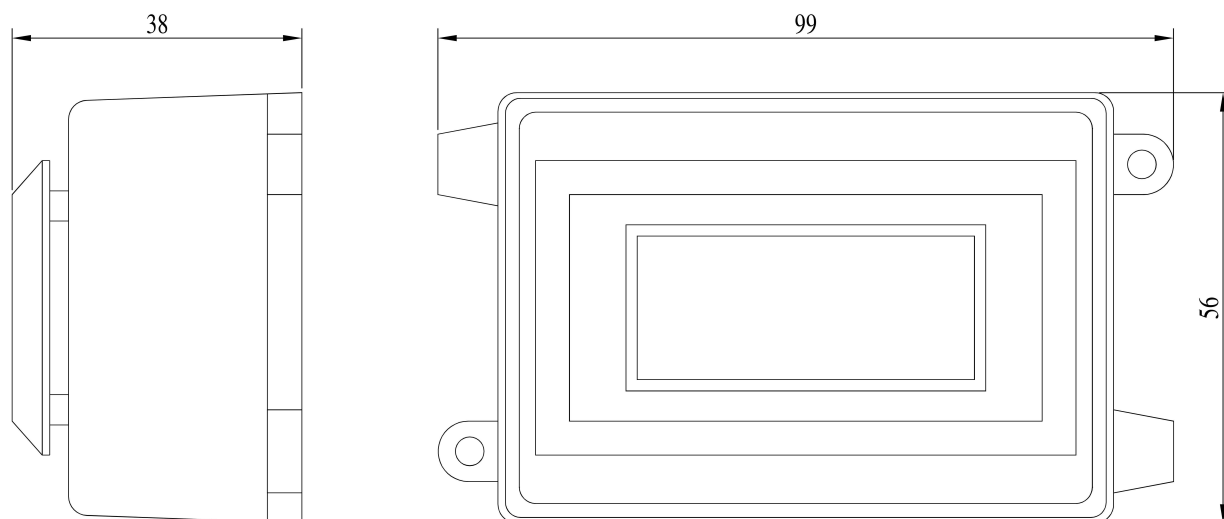
Рисунок 2б. Габаритные размеры изделия
