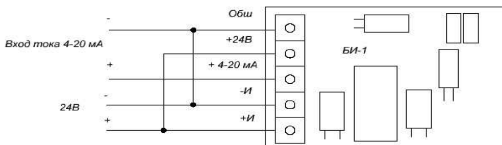
Рисунок 3. Подключение БИ-1. Вариант с одним источником питания
