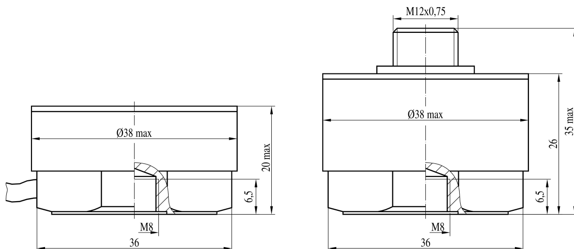
Рисунок 2. Габариты датчика
