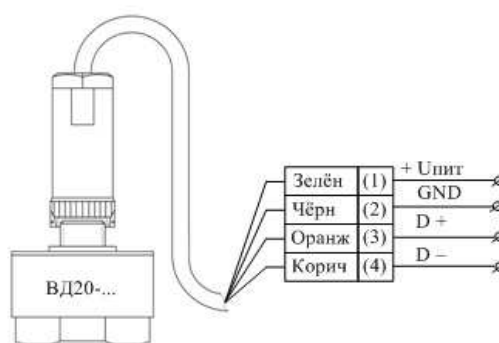
Рисунок 1. Схема подключения датчика с разъёмным кабелем.
