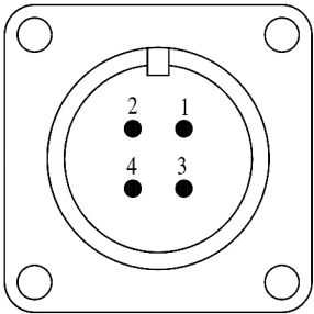
Разъем PC4ТВ датчика
